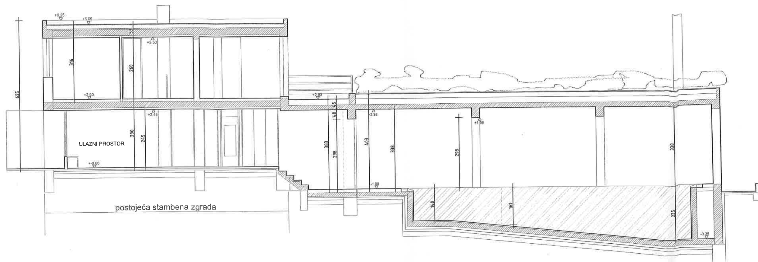
presjek 2-2
